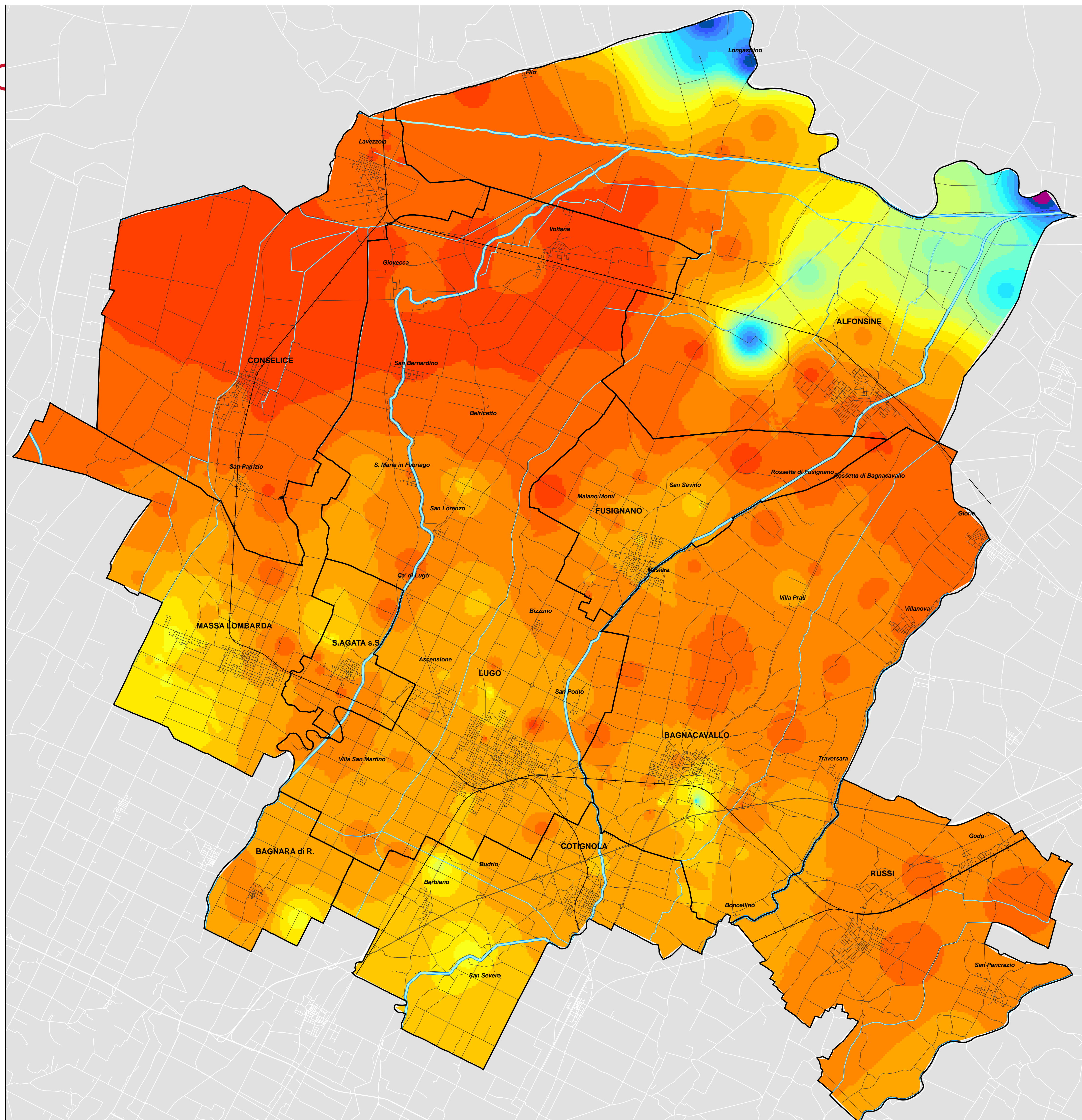
Tavola 35 (SNA19) - Resistenza alla punta da 6 a 10 mt di profondità (rif. Carta 1-3 elaborato specialistico "Geologia, ambiente, sismica")
